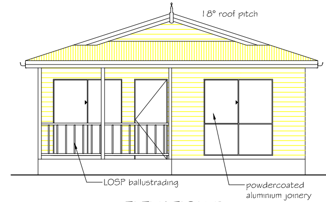
ELEVATION B
